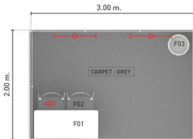
LAY-OUT-PLAN SCALE 1:50
